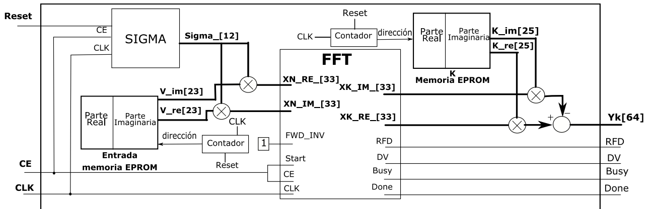
Figura 5. Diagrama de bloques de la TNLI.
