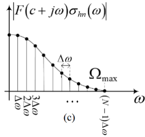
Figura 1. Discretización de F(c+j\omega)\sigma_m(\omega) muestreo RU.
